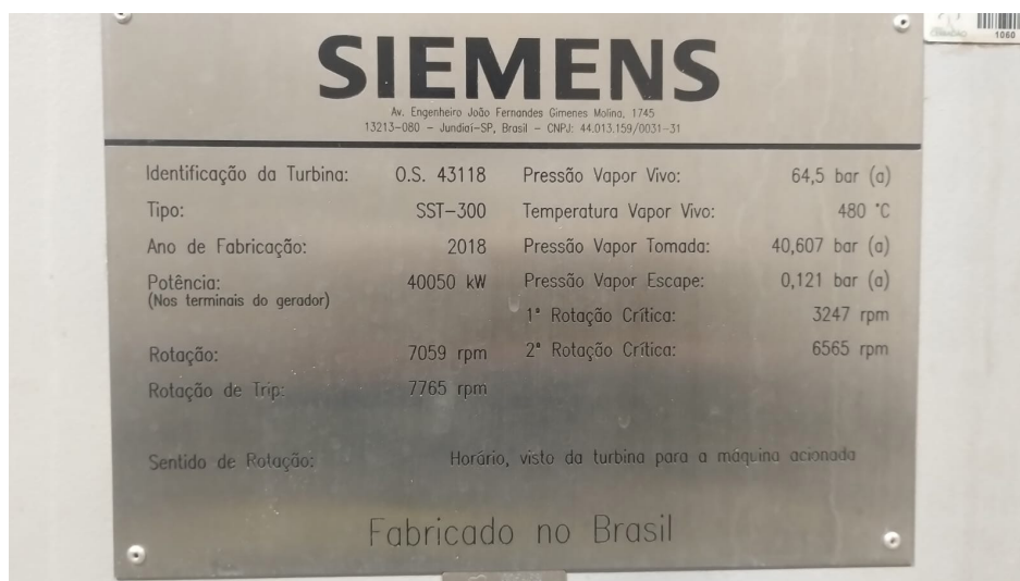
Turbine nº 3
