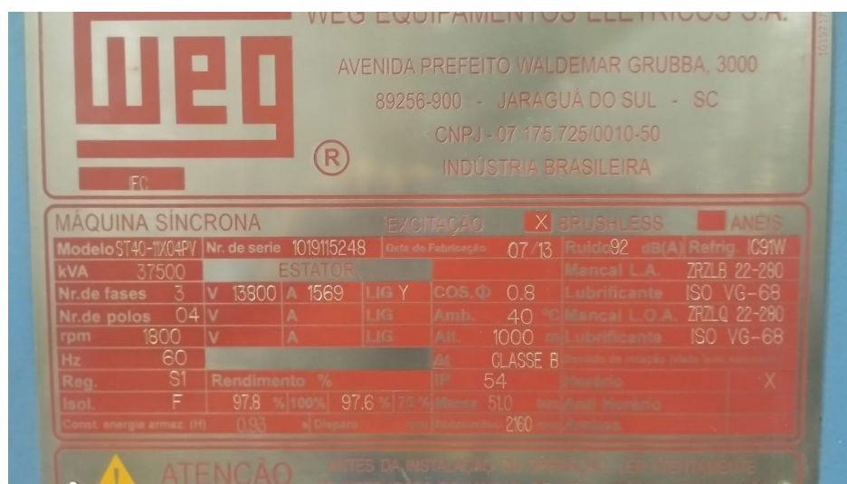
Alternator/ Generator nº 2
