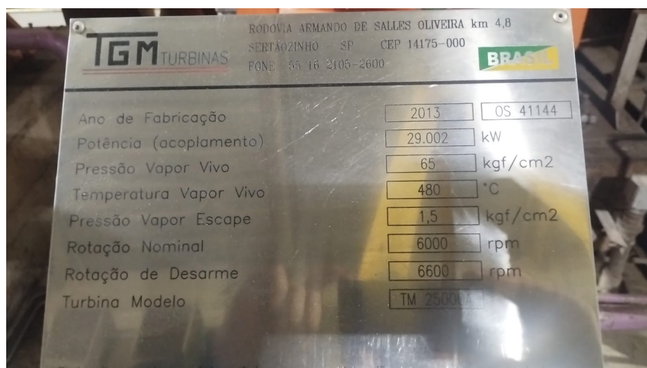
Turbine nº 1
